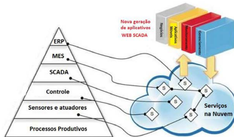
Figura 5. Sistema SCADA baseado na arquitetura SOA (LOJKA et al, 2016).
