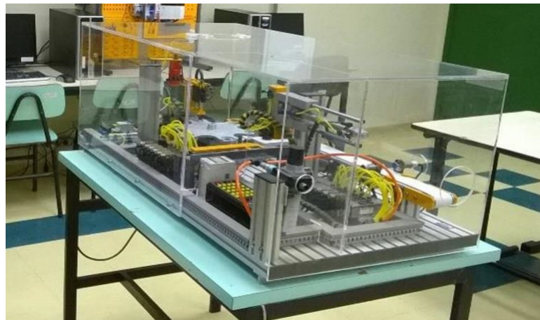
Figura 6. Célula de manufatura didática instalada no Campus São Paulo do IFSP.
