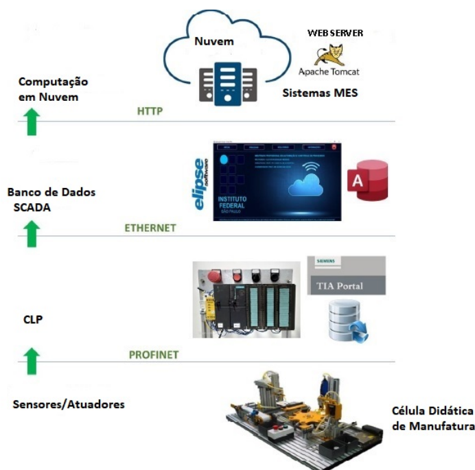
Figura 7. Arquitetura proposta para digitalização da célula didática de manufatura.
