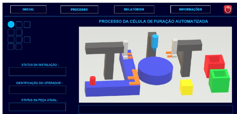
Figura 9. Tela do sistema de SCADA.
