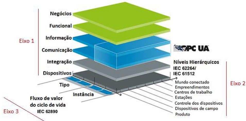
Figura 2. Arquitetura do Modelo de referência RAMI (SCHWEICHHART, 2016).
