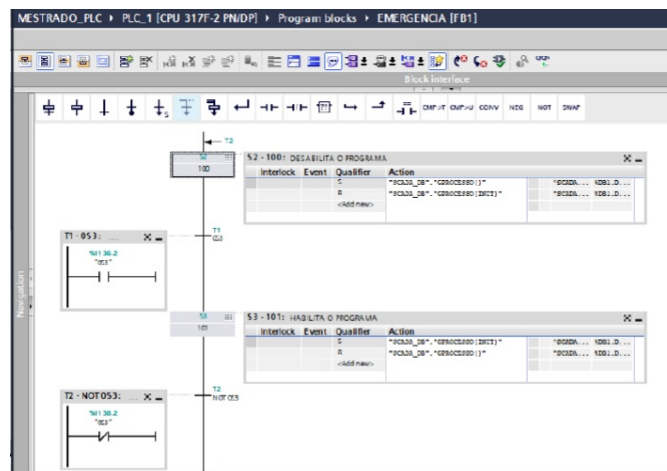
Figura 8. Linguagem Grafcet utilizada na programação do CLP.
